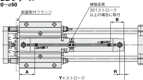
C-C'矢視図
