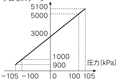
ZSE20BF-L(連成圧用) プロセスデータ
