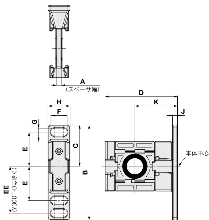
ブラケット付スペーサ
